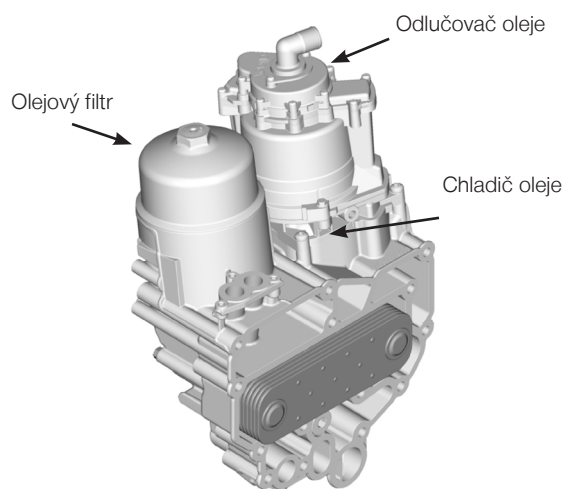
Obr. 2: Olejový modul Euro 6
